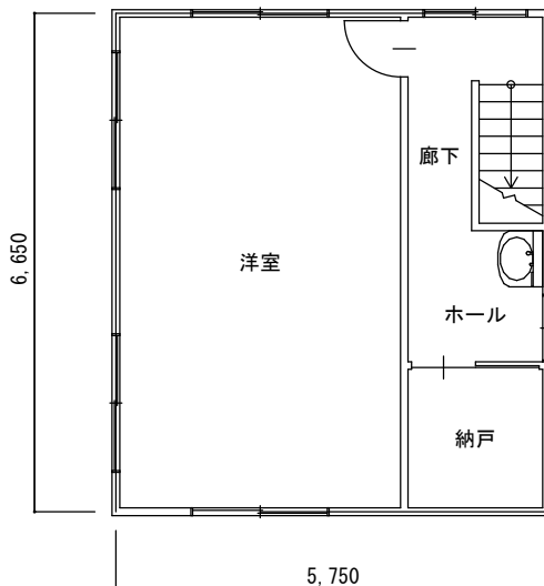
改修前 2階平面図
